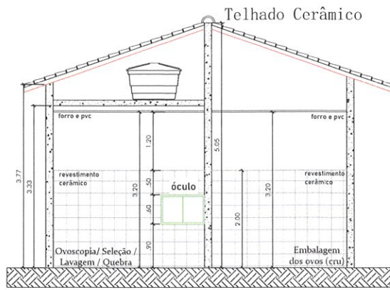
Corte AA ESCALA 1:75
