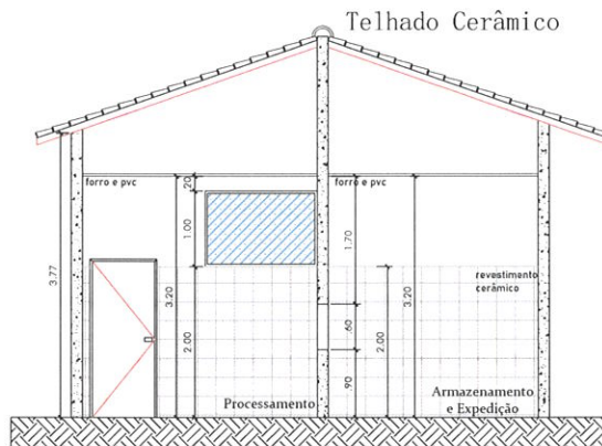
Corte BB ESCALA 1:75
