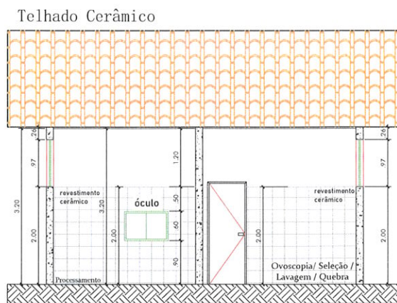
Corte CC ESCALA 1:75
