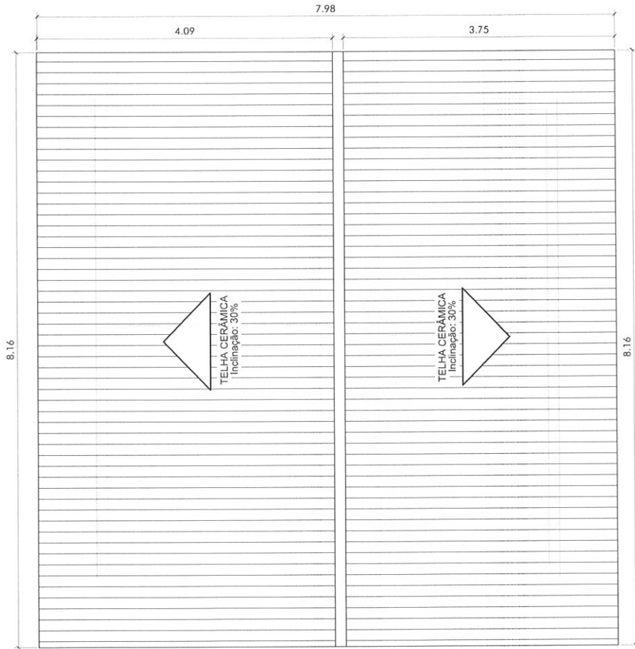
Planta de Cobertura ESCALA 1:75
