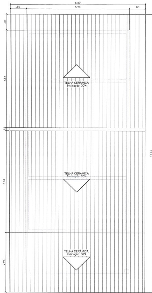
Planta de Cobertura ESCALA 1:50
